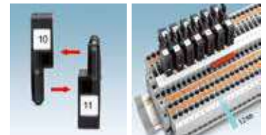
P-FU ...-5 sigorta fişi 5,2 mm genişlikte (2,5 mm 2 lik) ...TG ayrırma klemensleriyle kullanılabilir ve maksimum alan kazancı sağlar.
