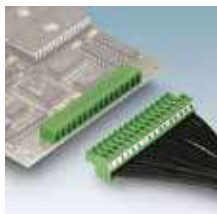
MC 1,5/...-G-3,81 & MC1,5/...-ST-3,81 (yatay soket + fiş)
