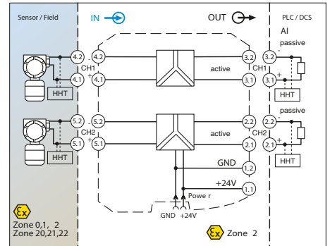
MACX MCR-EX-SL-RPSS-2I-2I için bağlantı şekli
