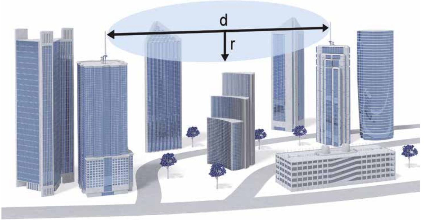
Şekil : Fresnel-Zone
